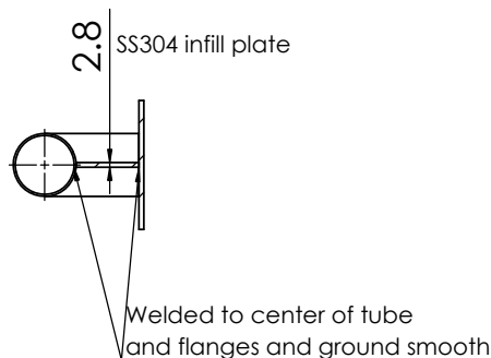
SECTION B-B SCALE 1 : 5
