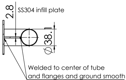
SECTION A-A SCALE 1 : 5
